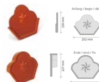
ukončení hřebenáče
