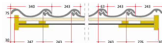
Taška ukončovací (s dvojistou naválkou)
