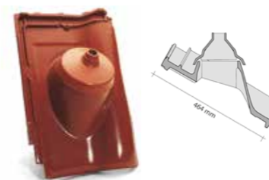
anténní komplet: prostupová taška s pryžovým nástavcem - hmotnost tašky cca: 4,3 kg - pryžový nástavec cca: 0,1 kg - hmotnost 1 ks cca: 4,4 kg
