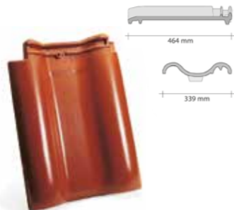
taška s dvojitou návalkou
